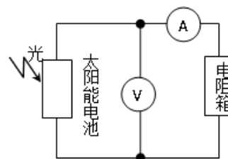
测量太阳能电池输出特性
